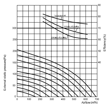
HRS-PRO500
