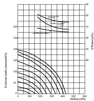
HRS-PRO350
