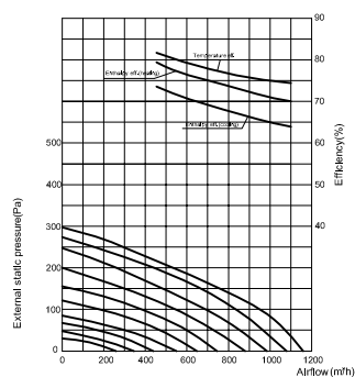
HRS-PRO1000
