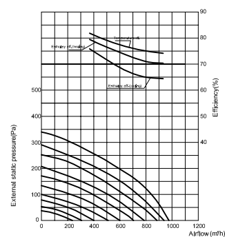
HRS-PRO800
