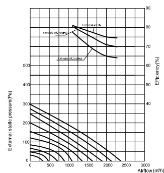
HRS-PRO2000
