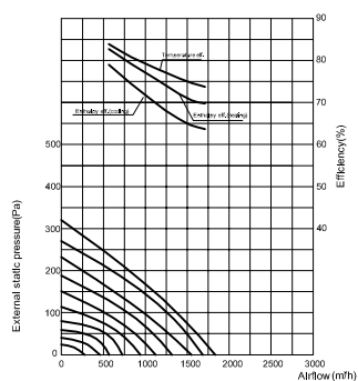
HRS-PRO1500
