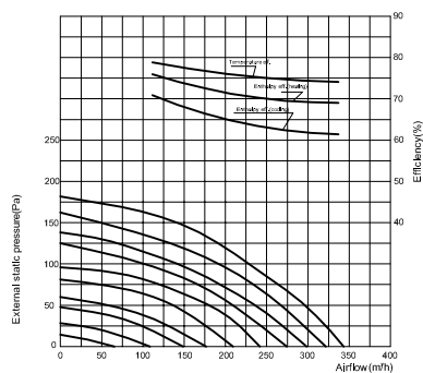
HRS-PRO250
